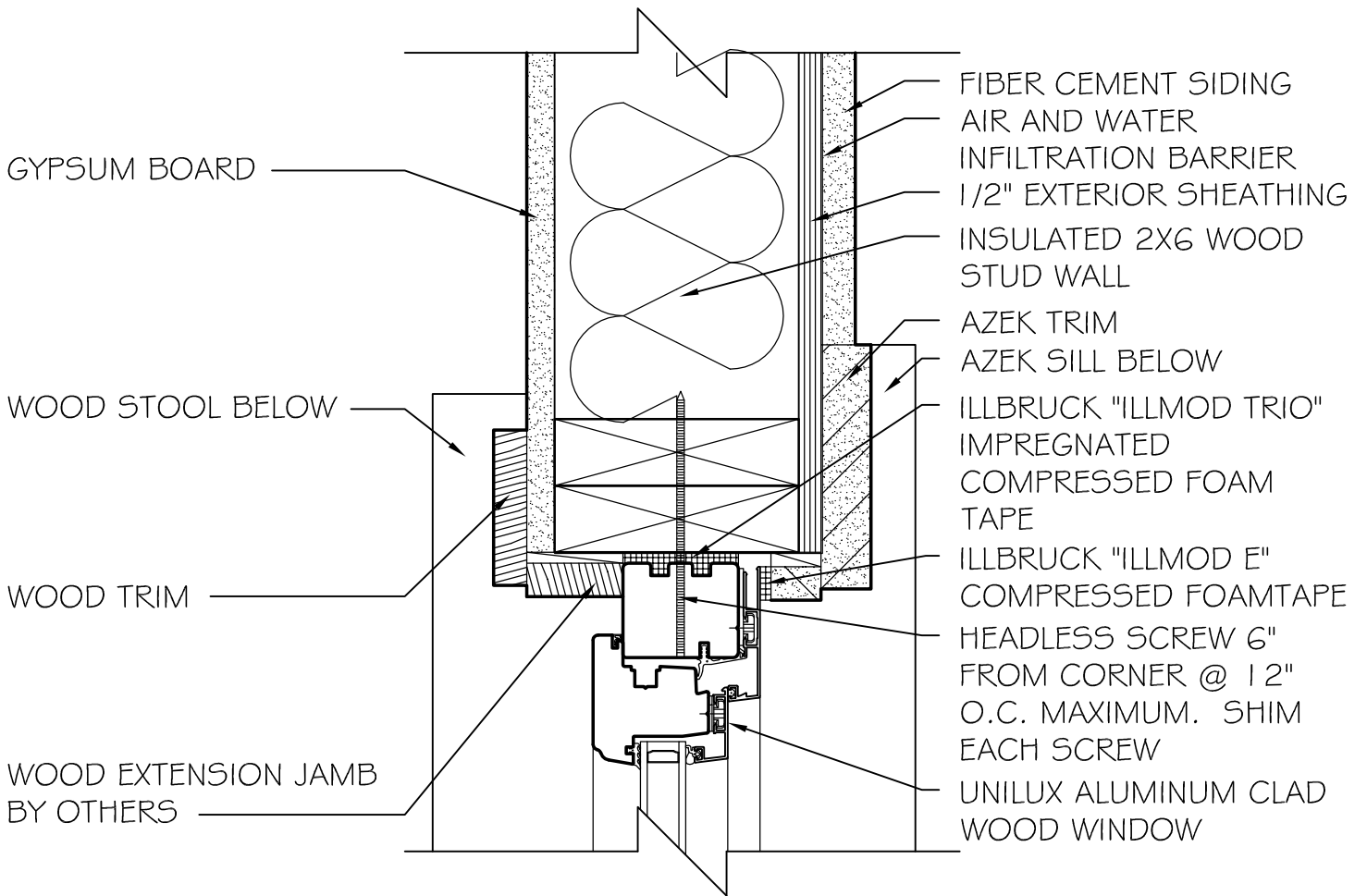
MID JAMB DETAIL SCALE: 3" = 1'-0"
