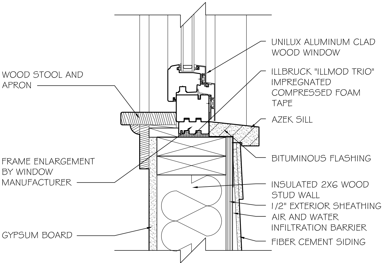
MID SILL DETAIL SCALE: 3" = 1'-0"
