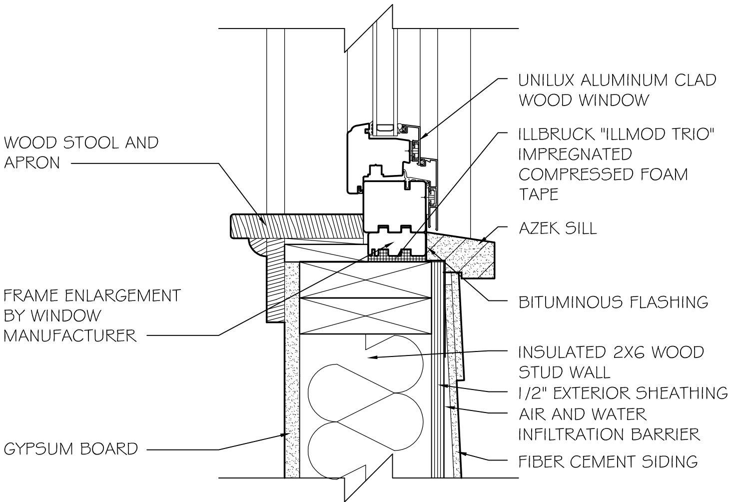
OUTBOUND SILL DETAIL SCALE: 3" = 1'-0"
