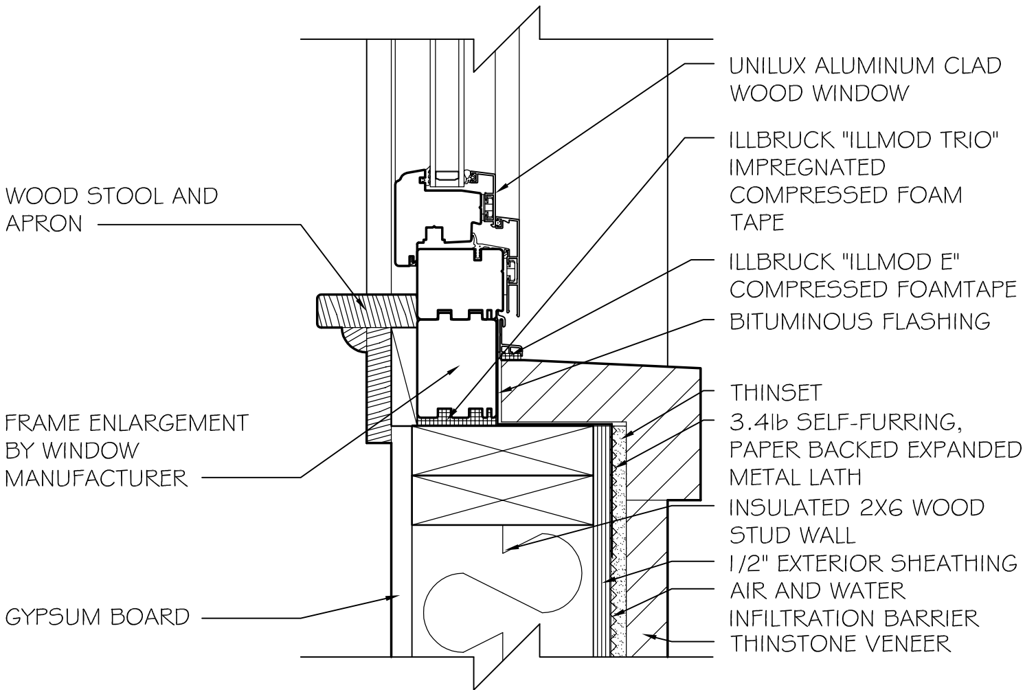
INBOUND SILL DETAIL SCALE: 3" = 1'-0"
